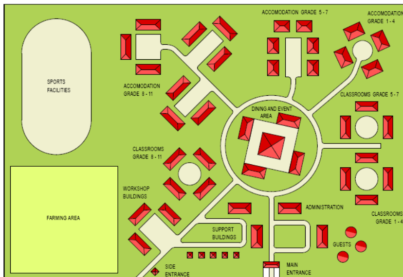
Abb. 1: Lageplan der Schule, Entwurf. Die Anordnung der Gebäude und Areale bezieht sich hier noch auf ein Grundstück mit den Abmessungen ca. 500 m x 400 m und muss nun den neuen Gegebenheiten (ca. 700 m x 300 m) angepaßt werden.
